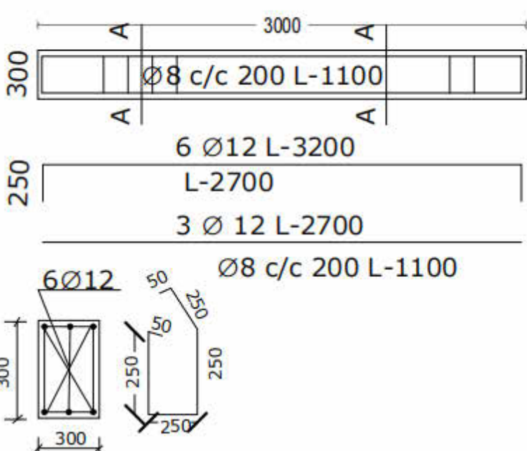
SECTION A-A SCALE 1:25
