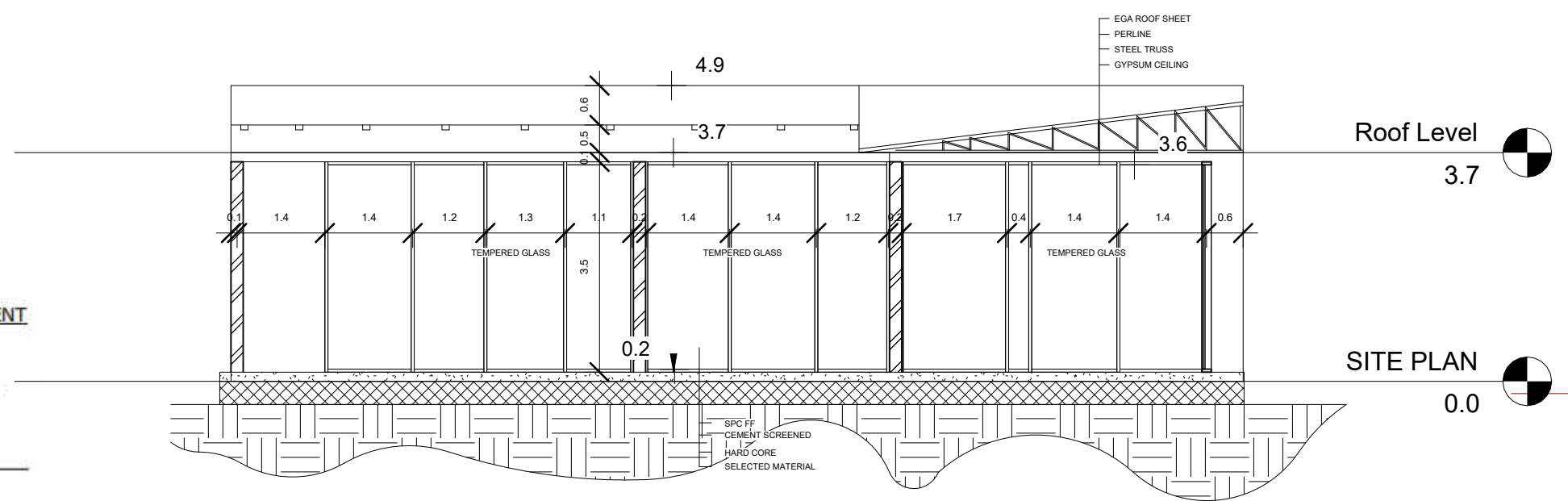
7 SECTION X 1 : 100
